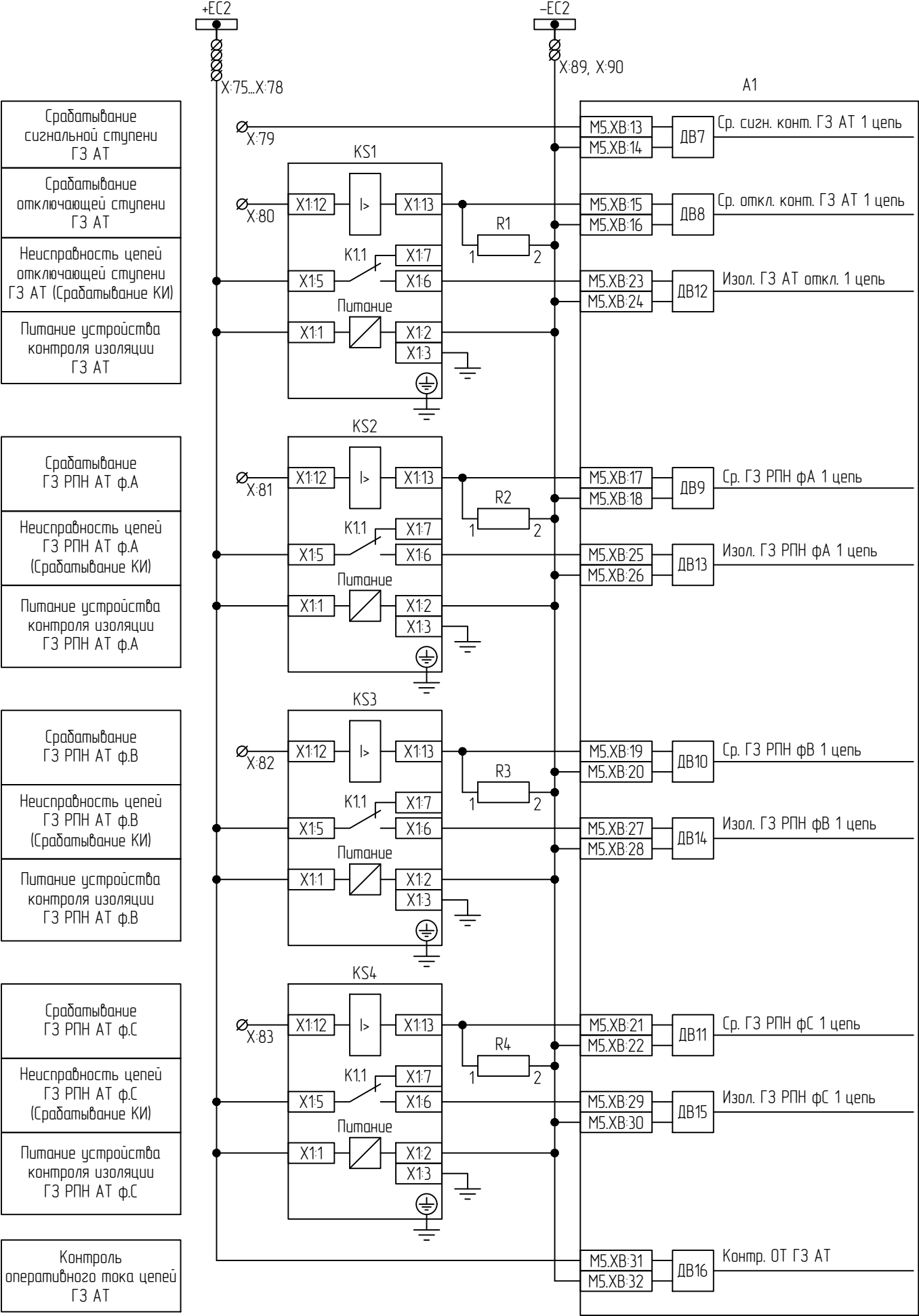
Цепи оперативного тока ГЗ АТ А1
